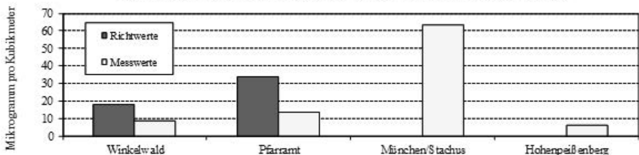
Mittlere Stickstoffdioxid-Konzentration im Zeitraum 14.12.2012 bis 14.02.2014
